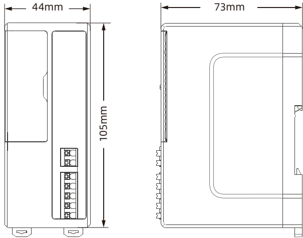
中继器尺寸
