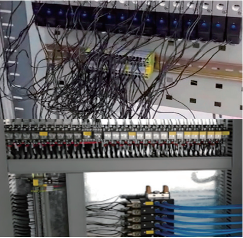
传统阀组接线
