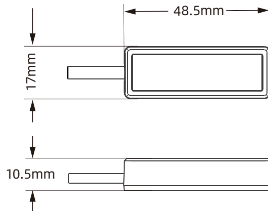
终端尺寸
