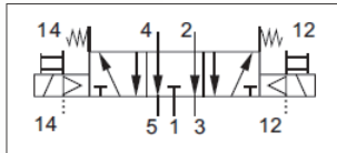
三位五通中泄
