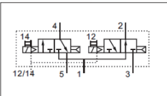
双两位三通NC/NO
