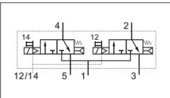
双两位三通NC (弹簧复位, 适用于负压)
