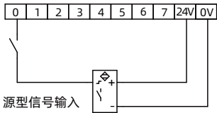
源型信号输入
