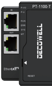
总线适配器
