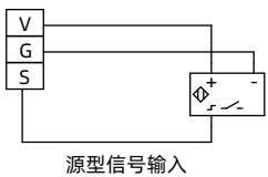
源型信号输入
