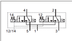
双两位三通NC (适用于正压)
