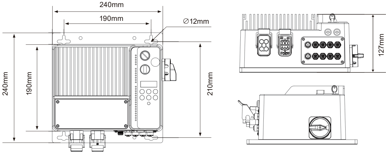
航插版:0.75-5.5kw
