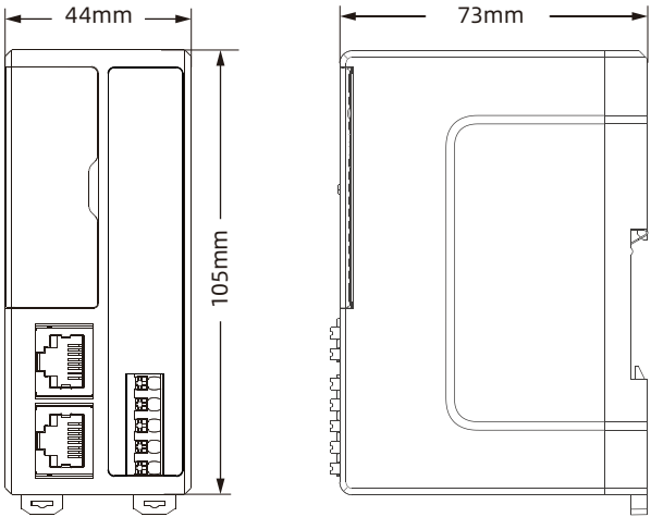
适配器尺寸
