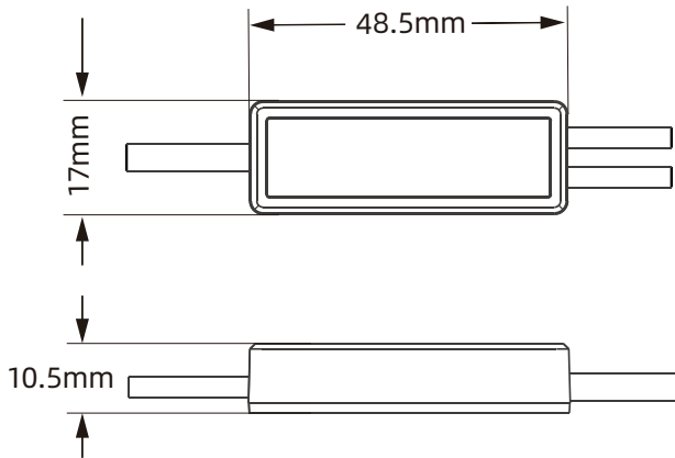
2点从站尺寸
