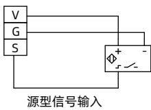
源型信号输入
