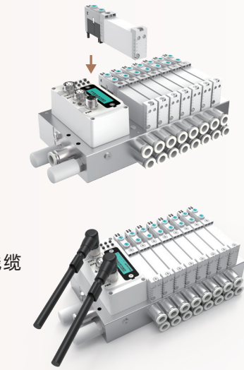
EV-FD阀岛接线
