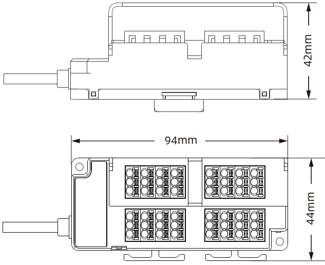
16点从站尺寸
