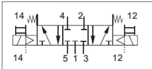
三位五通中封
