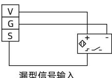
漏型信号输入
