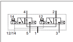
双两位三通NO
