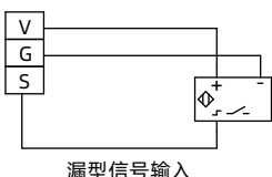
漏型信号输入
