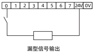
漏型信号输出
