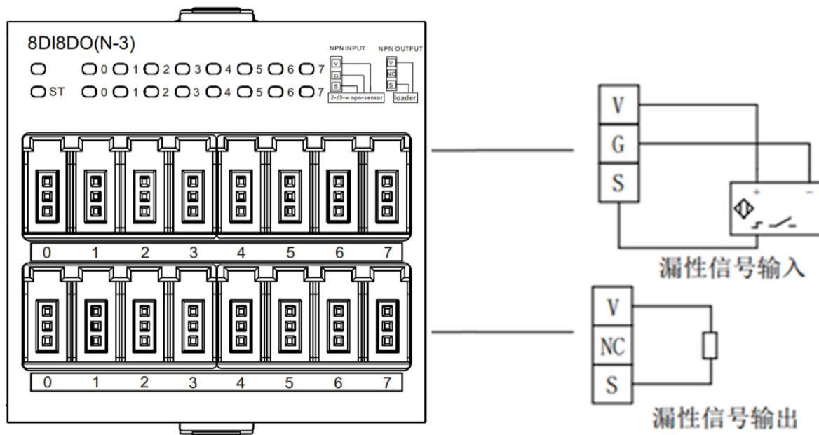
8DI8DO(N-3)
