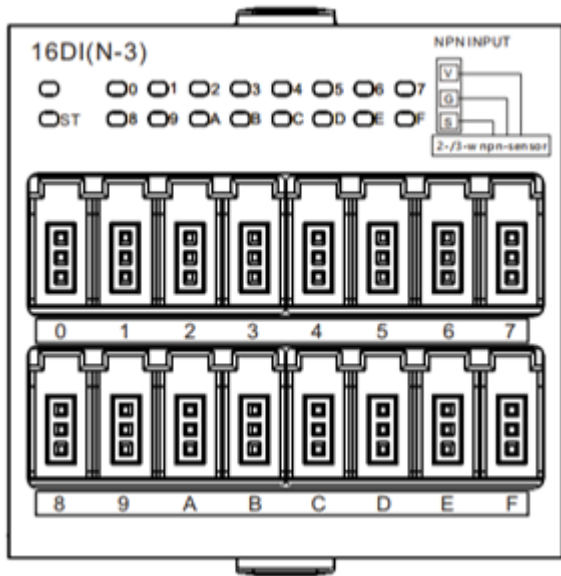
16DI(N-3)
