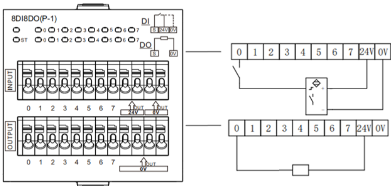
8DI8DO(P-1)
