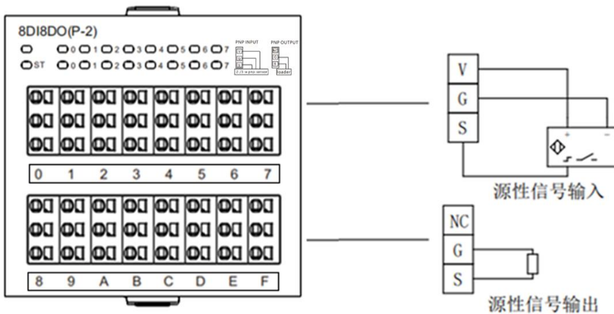
8DI8DO(P-2)
