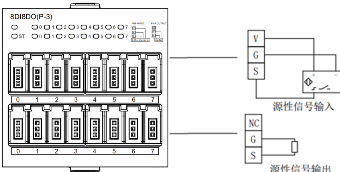
8DI8DO(P-3)
