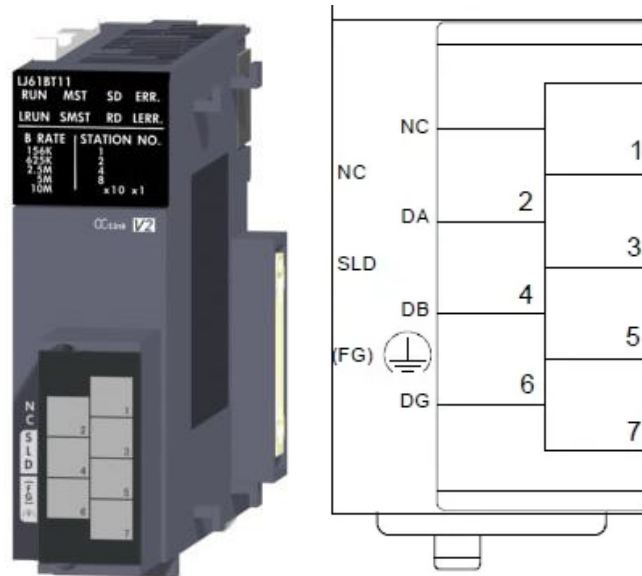
硬件连接图
