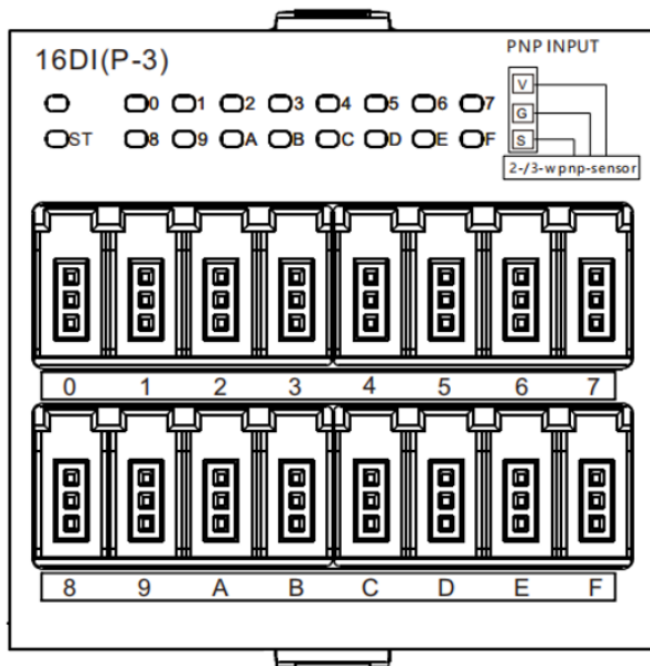
16DI(P-3)
