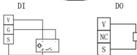
16DIO(N-2)
