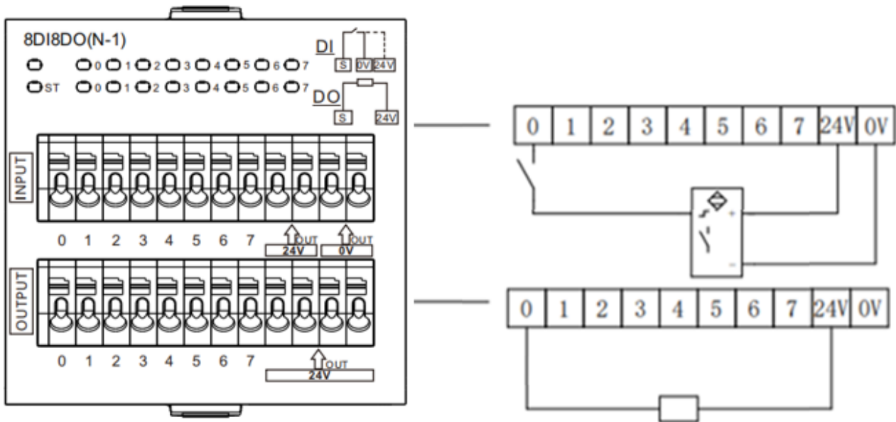
8DI8DO(N-1)
