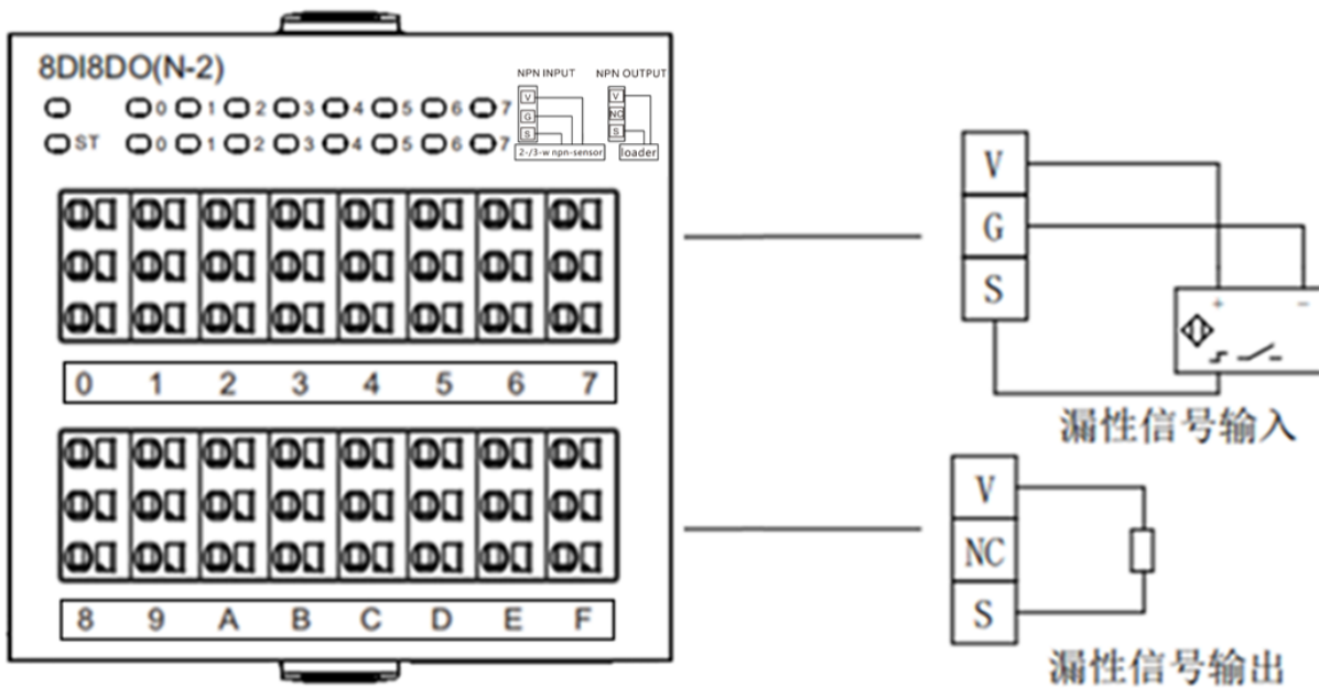
8DI8DO(N-2)
