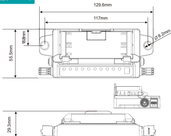
内驱 (RD-UD20)
