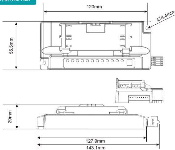
外驱 (RD-ND)
