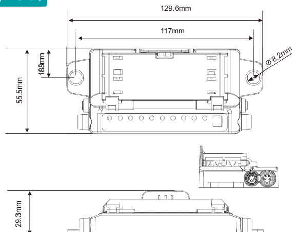
内驱 (RD-UD67)
