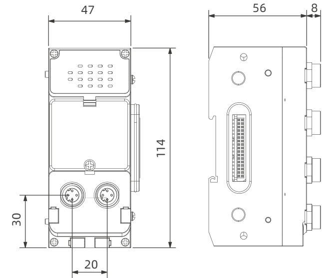
通讯模块尺寸图
