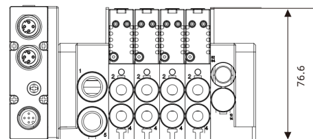
紧凑型阀岛尺寸图 (2 系)
