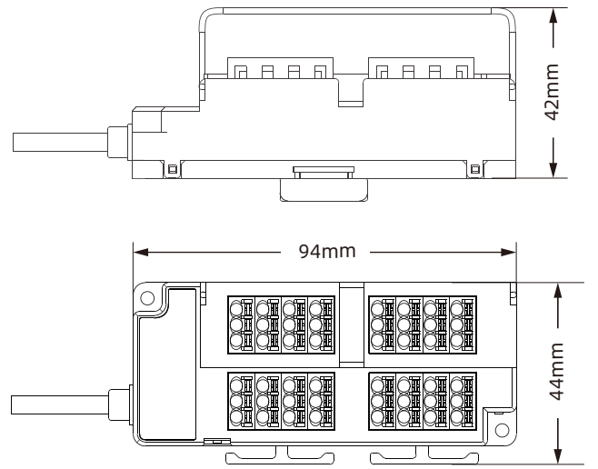
16点从站尺寸
