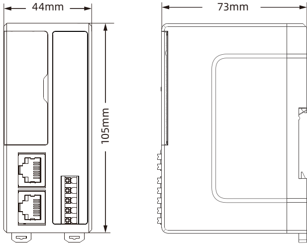
适配器尺寸
