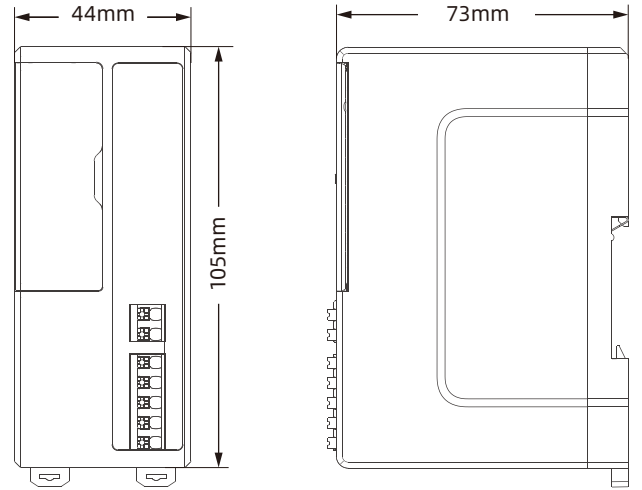
中继器尺寸
