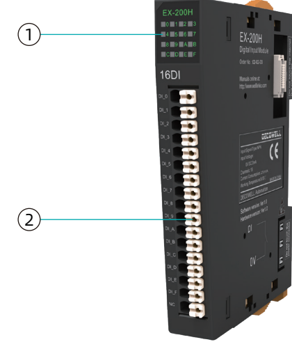
① 状态指示灯 ② 接线端子
