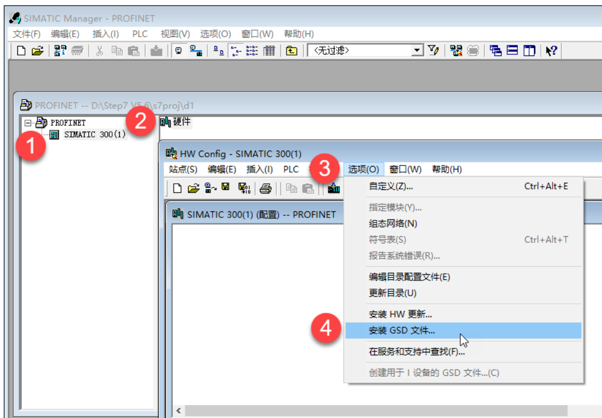
图 4-3-2 安装 GSD 文件
