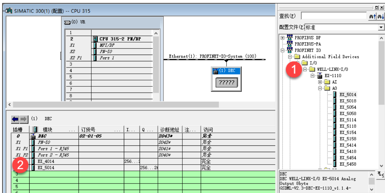
图 4-3-10 添加 I/O 模块
