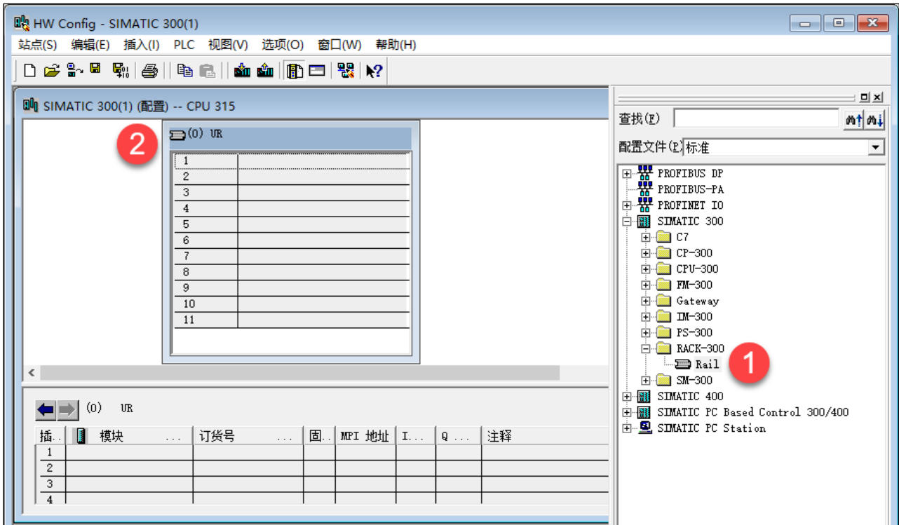
图 4-3-6 添加机架 Rail
