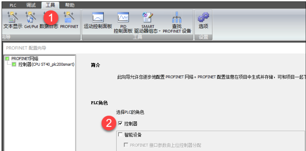
图 4-2-4 选择 PLC 角色
