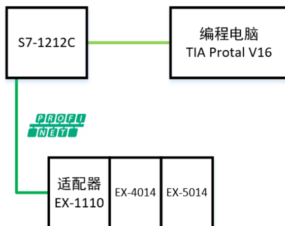
图 4-1-1 通讯连接图
