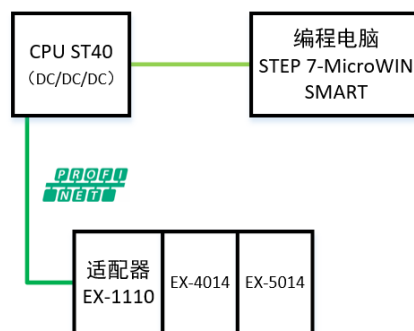
图 4-2-1 通讯连接图
