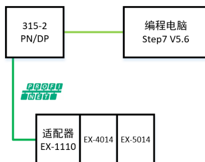
图 4-3-1 通讯连接图
