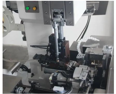
端子机
