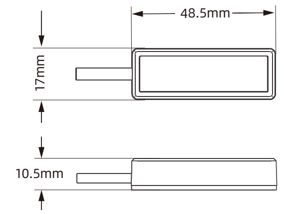
终端尺寸
