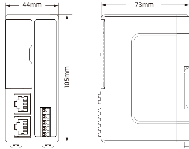
适配器尺寸
