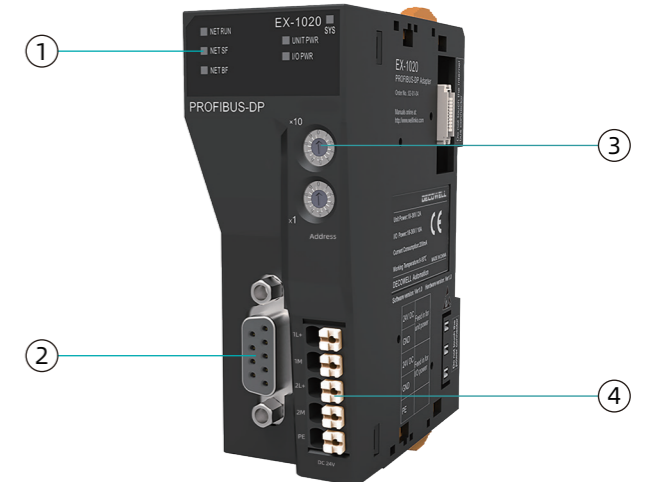
① 状态指示灯 ② 通讯接口 ③ 适配器拨码设置 ④ 电源端口
