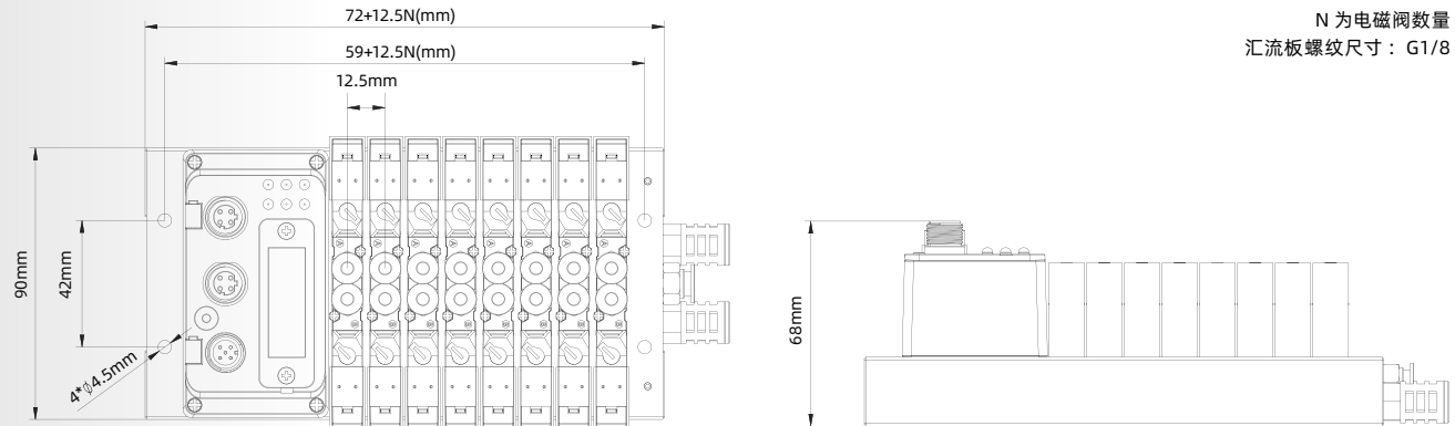
匹配 EV-1 电磁阀
